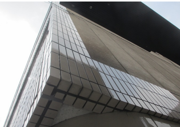
■ 工事名:都内ビル外壁改修工事 ■ 施工年:2020年 ■ 施工場所:東京都 ■ 施工数量:109㎡ ■ 目的:タイルおよびモルタル目地表面保護
