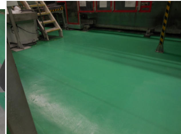
■ 工事名:ユニ・チャームペットケア(株)三重工場床面塗装工事 ■ 施工年:2014年 ■ 施工場所:三重県 ■ 施工数量:400㎡ ■ 目的:コンクリート床塗り替え・防塵・防滑(USCPモルタル併用)
