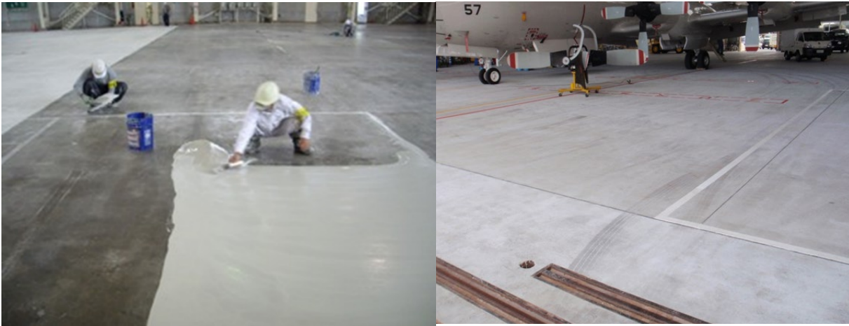
■ 工事名:第1格納庫施設コンクリート床塗装工事 ■ 施工年:2010年 ■ 施工場所:沖縄県 ■ 施工数量:3220㎡ ■ 目的:不陸調整(T&C防食併用)
