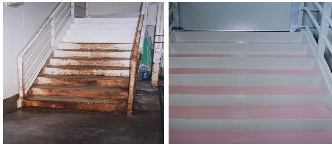
■ 工事名:倉庫鉄骨階段塗装工事 ■ 施工年:2011年 ■ 施工場所:東京都 ■ 施工数量:10㎡ ■ 目的:鉄骨階段(既設)補修・防錆
